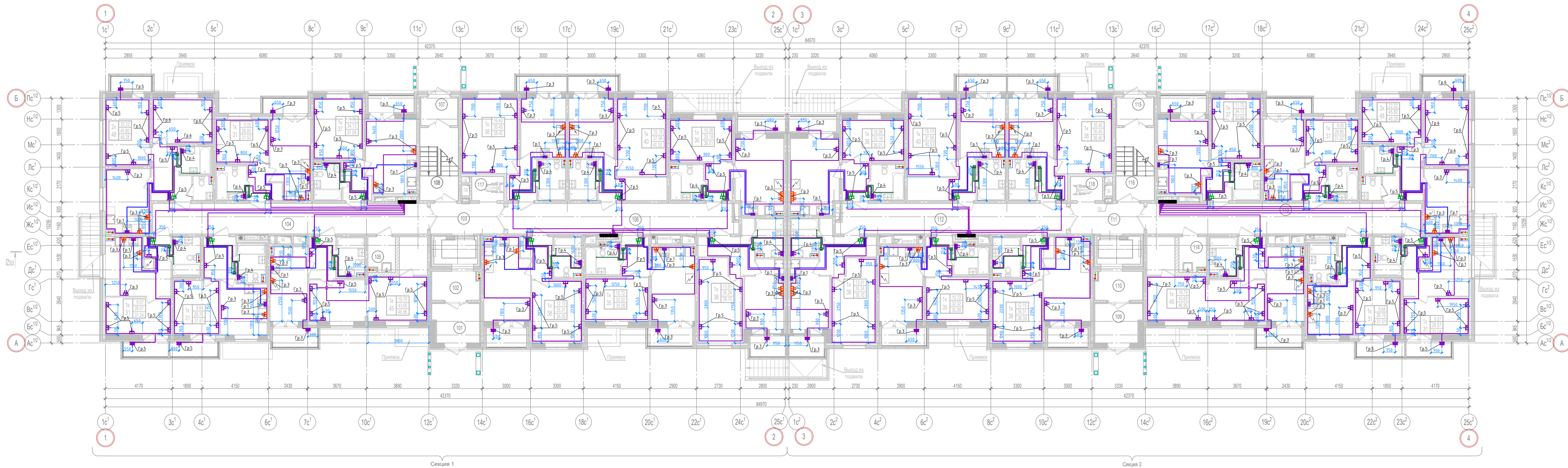
План 1 этажа
